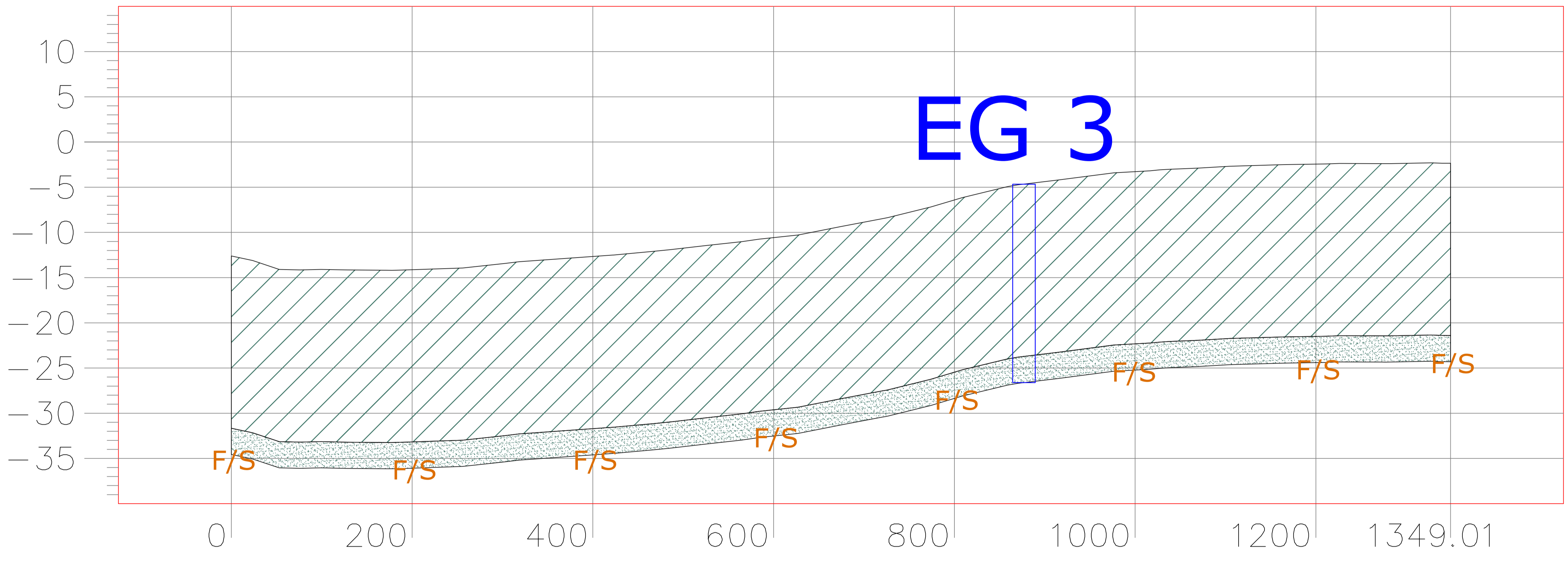
PERFIL EG3 ESCALA HORIZONTAL 1 : 1000 ESCALA VERTICAL 1 : 100
