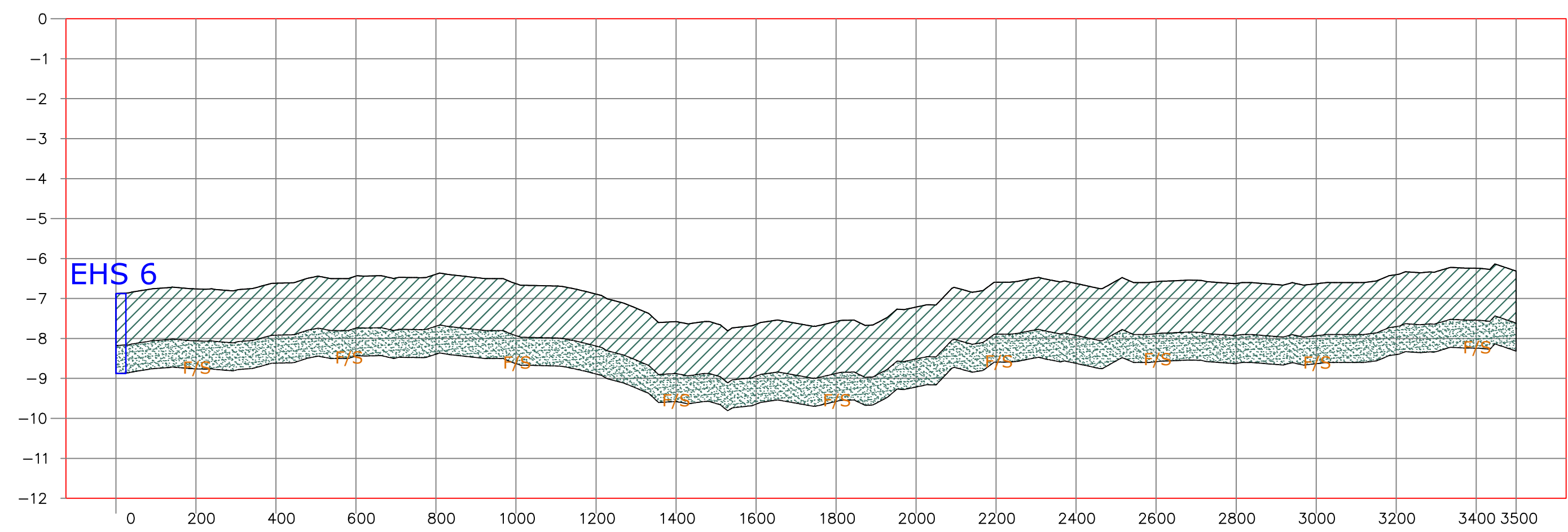
PERFIL EHS6- EHS8 (Tramo1) ESCALA HORIZONTAL 1 : 1000 ESCALA VERTICAL 1 : 10
