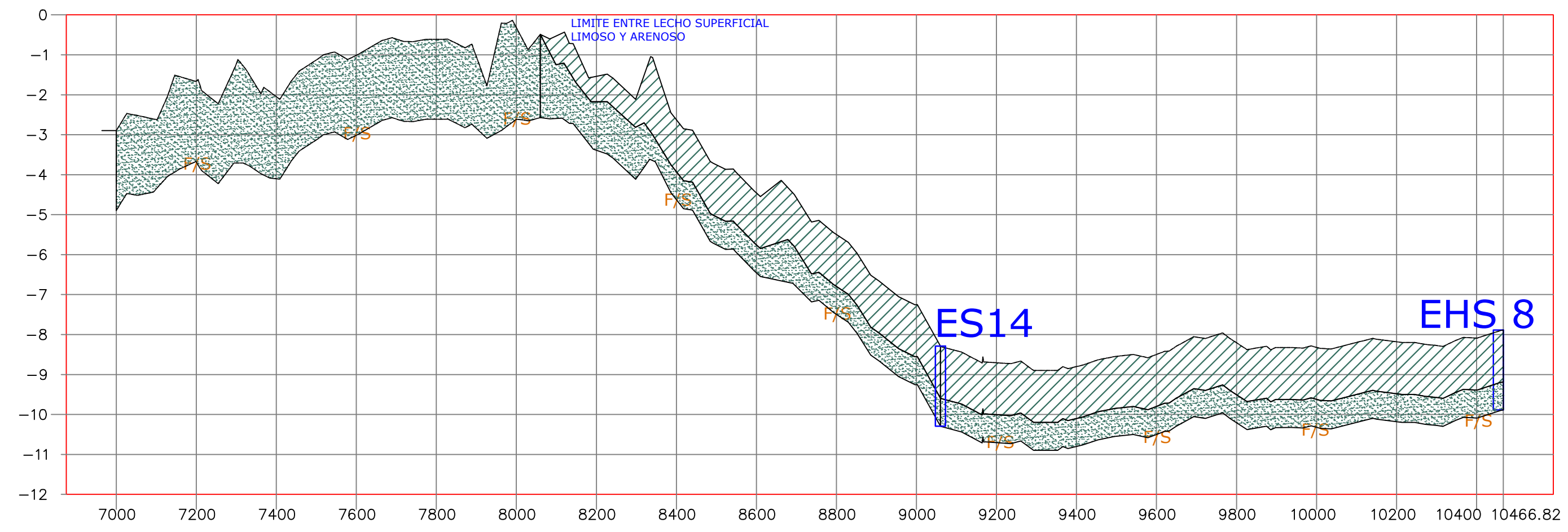
PERFIL EHS6- EHS8 (Tramo3) ESCALA HORIZONTAL 1 : 1000 ESCALA VERTICAL 1 : 10
