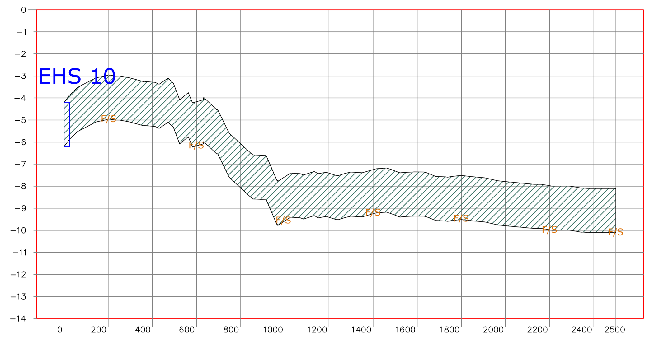
PERFIL EHS10 - EHS11 (Tramo1) ESCALA HORIZONTAL 1 : 1000 ESCALA VERTICAL 1 : 10
