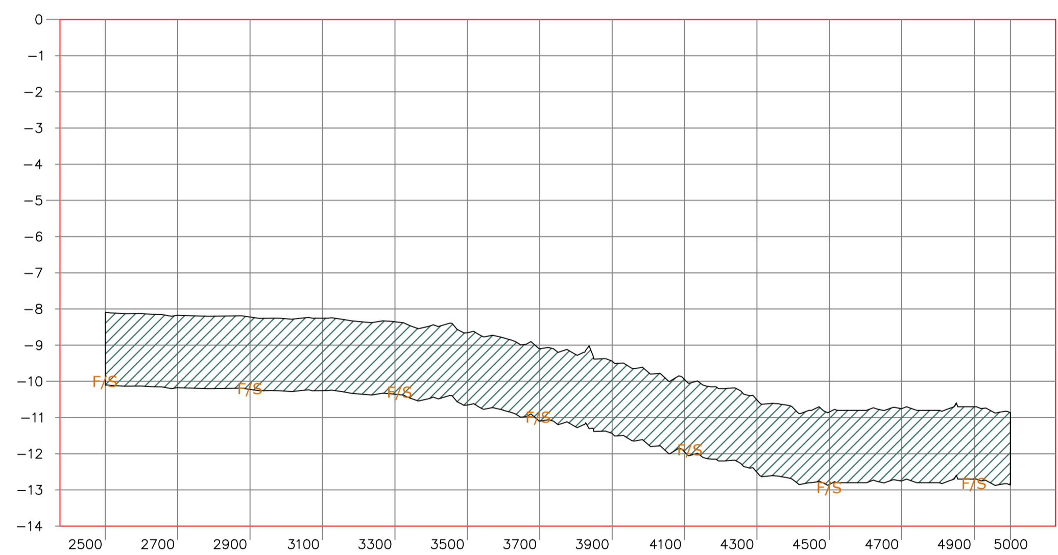
PERFIL EHS10 - EHS11 (Tramo2) ESCALA HORIZONTAL 1 : 1000 ESCALA VERTICAL 1 : 10
