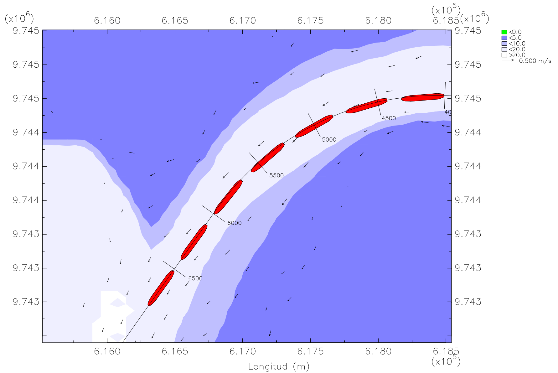
Z3T3 Trayectoria del barco portacontenedores post-panamax y corriente en reflujos
