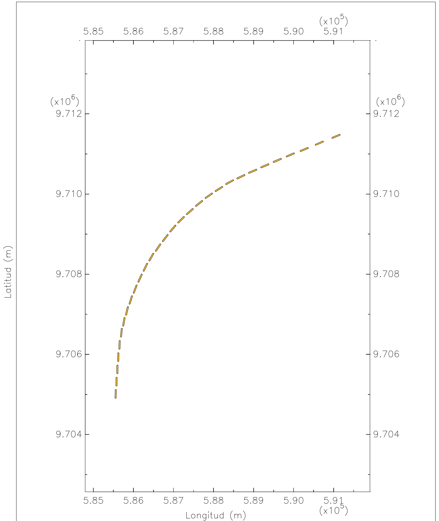
Zona 2 Trayectoria del barco granelero en reflujos
