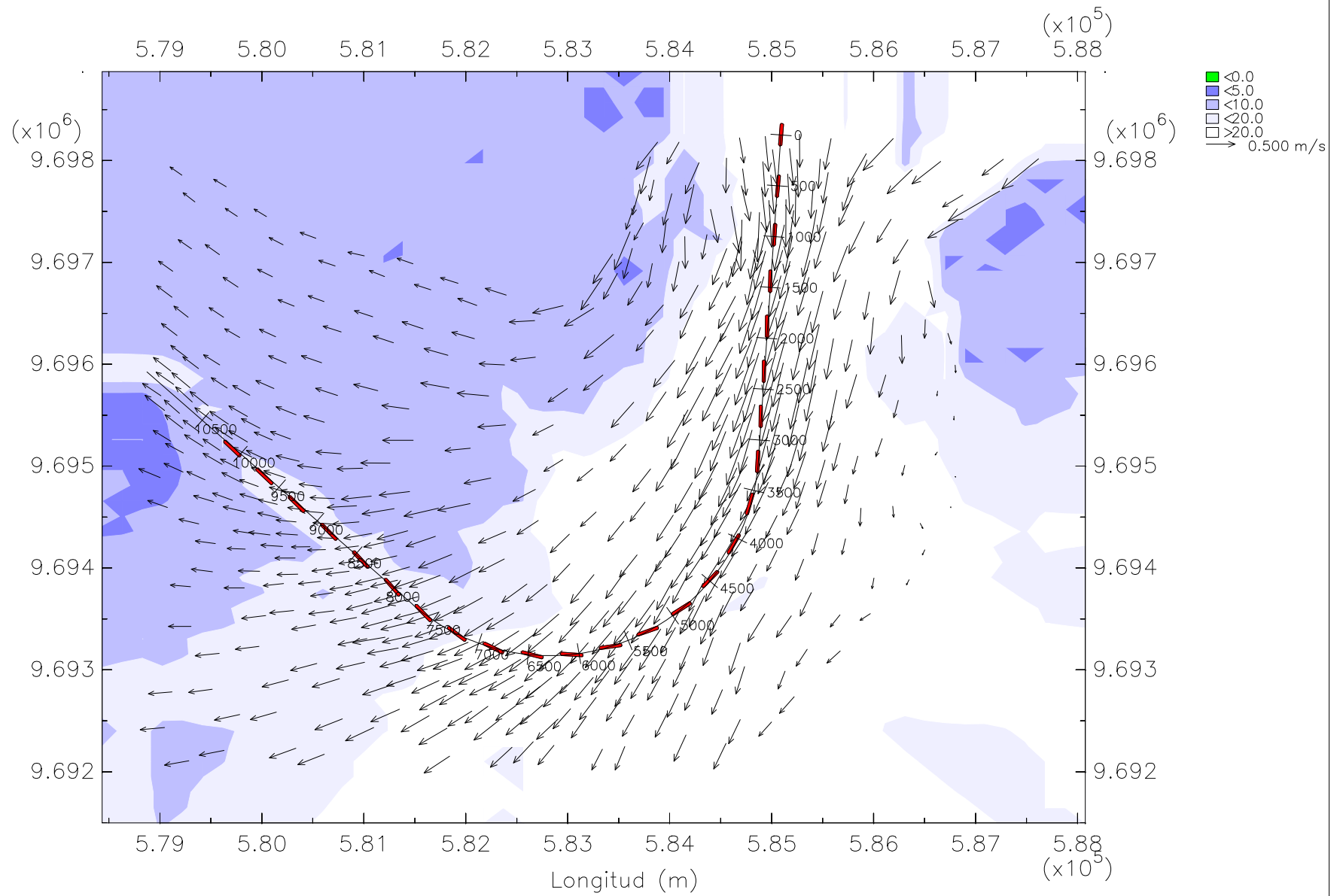
Zona 1 Trayectoria del barco granelero con corriente en refluo
