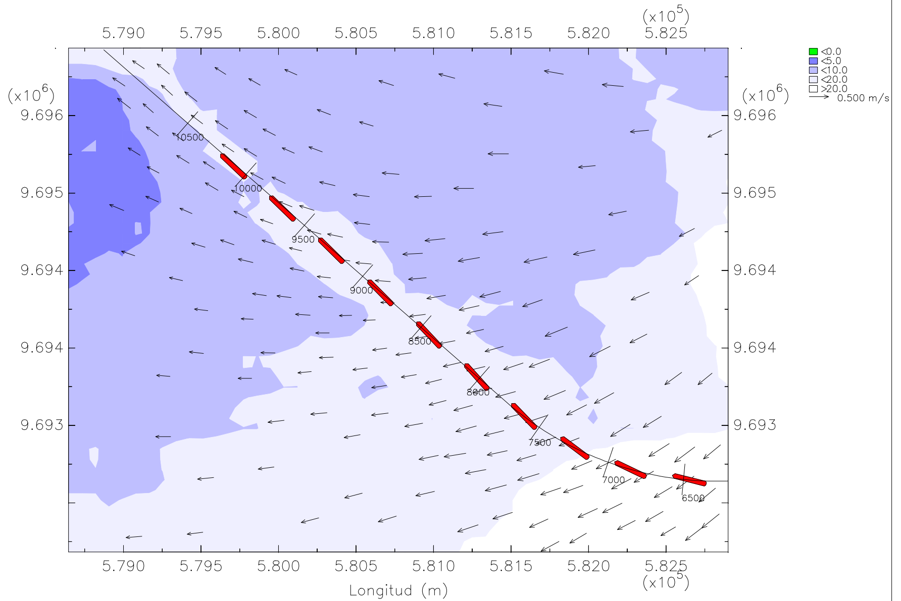
Z1T3 Trayectoria del barco granelero con corriente en reflujó
