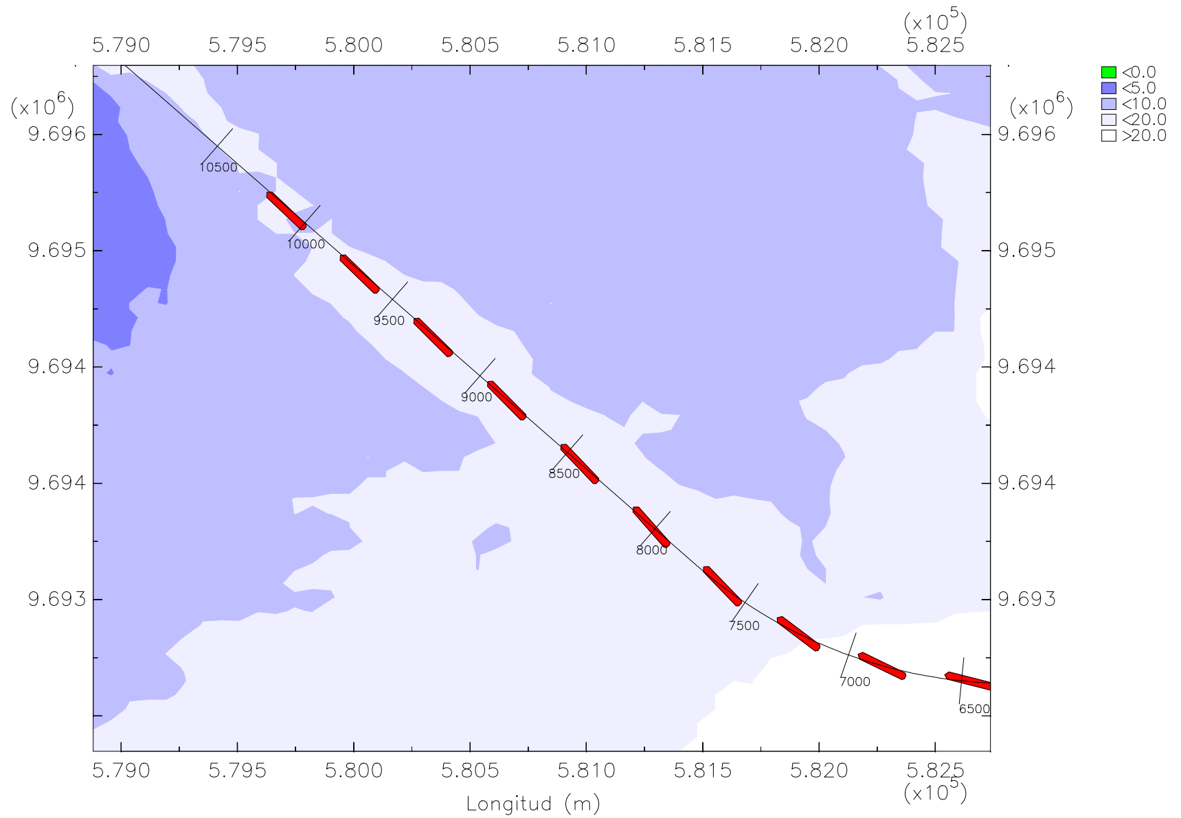
Z1T3 Trayectoria del barco granelero en refluo con profundidad
