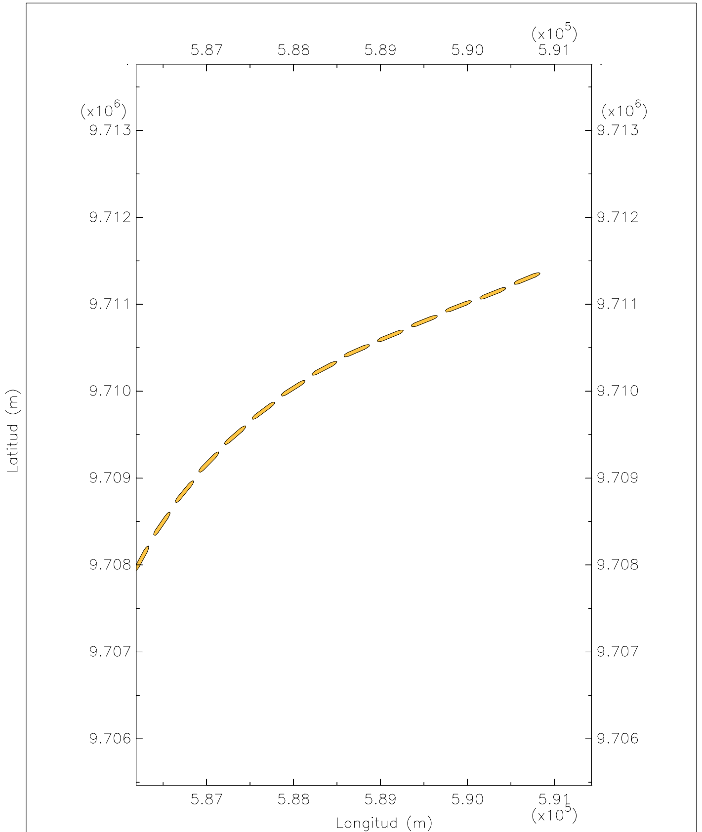
Z2T2 Trayectoria del barco en flujo
