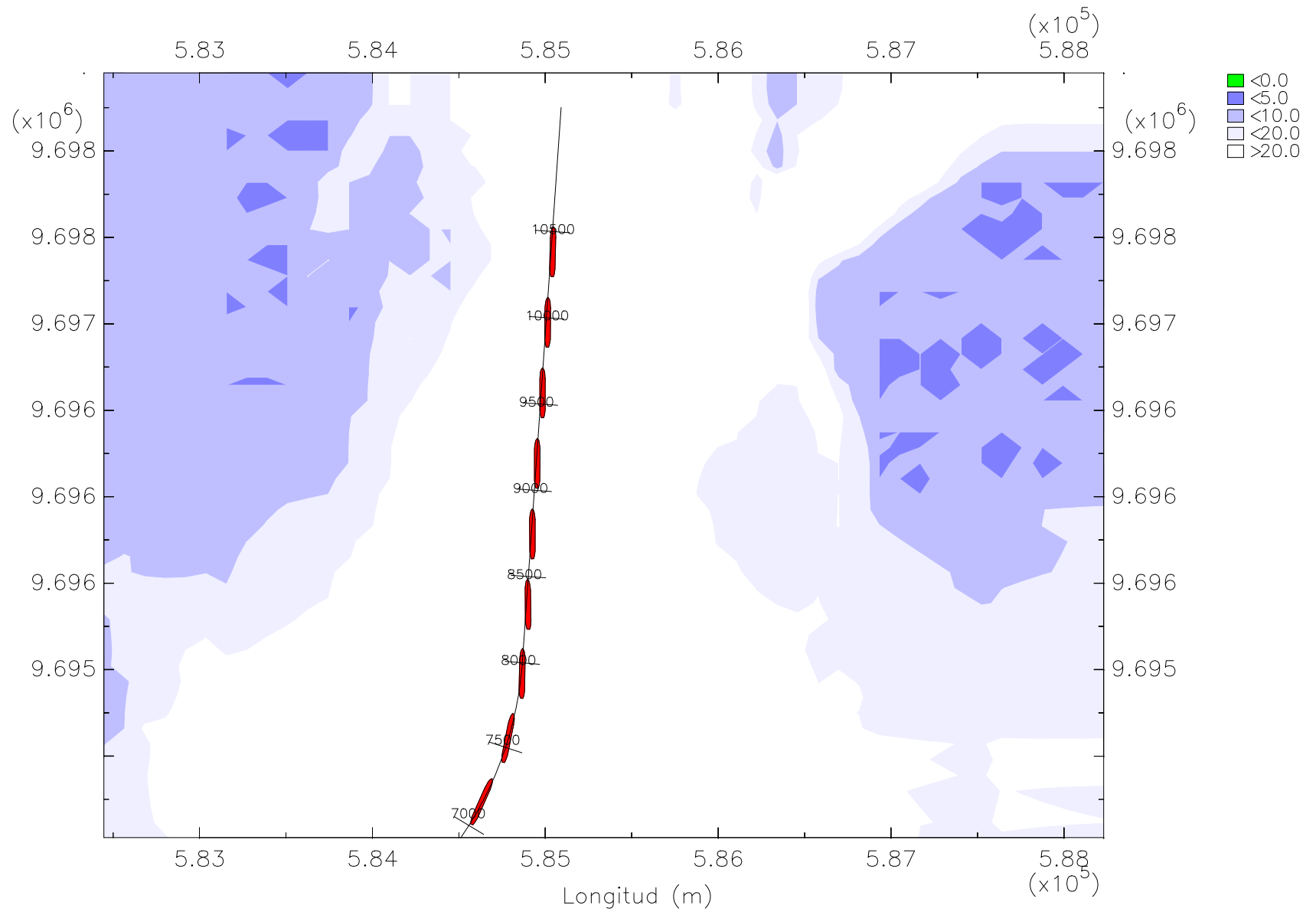
Z1T3 Trayectoria del barco portacontenedores panamax con profundidad
