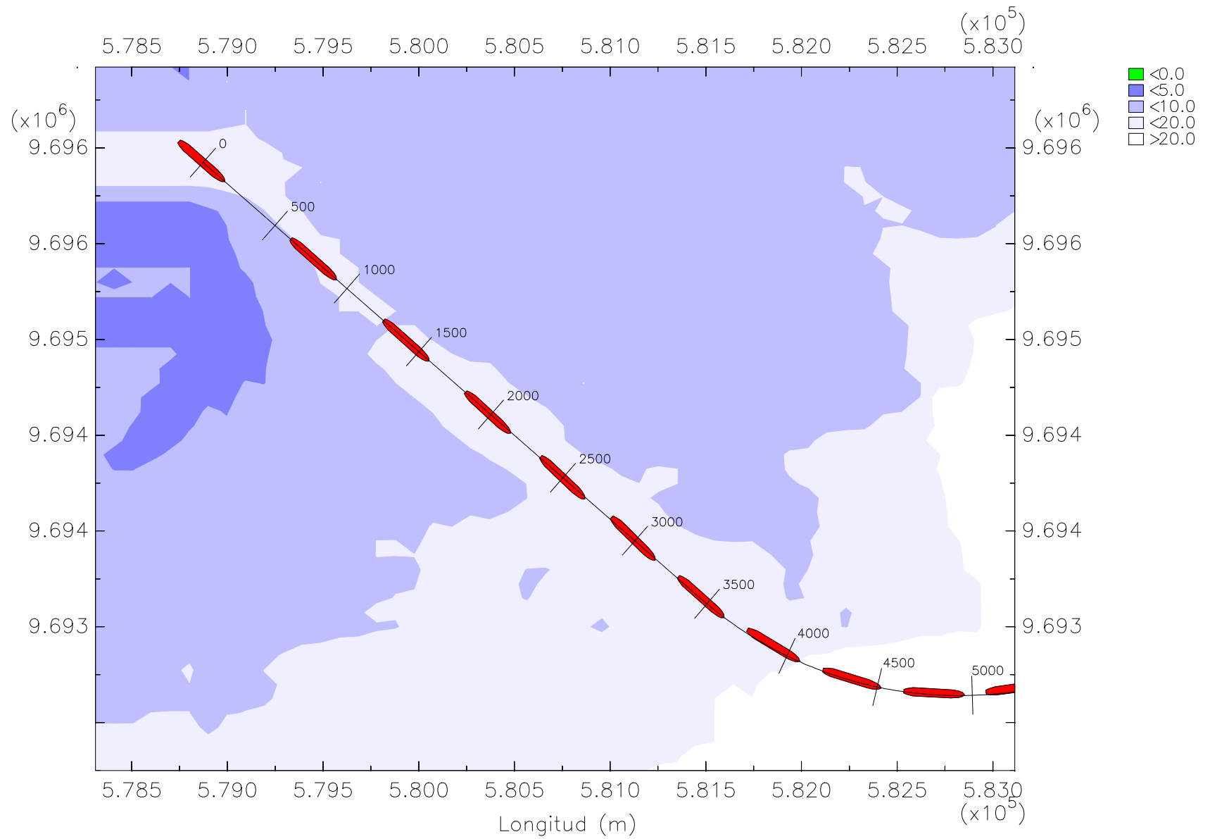
Z1T1 Trayectoria del barco portacontenedores post-panamax con profundidad
