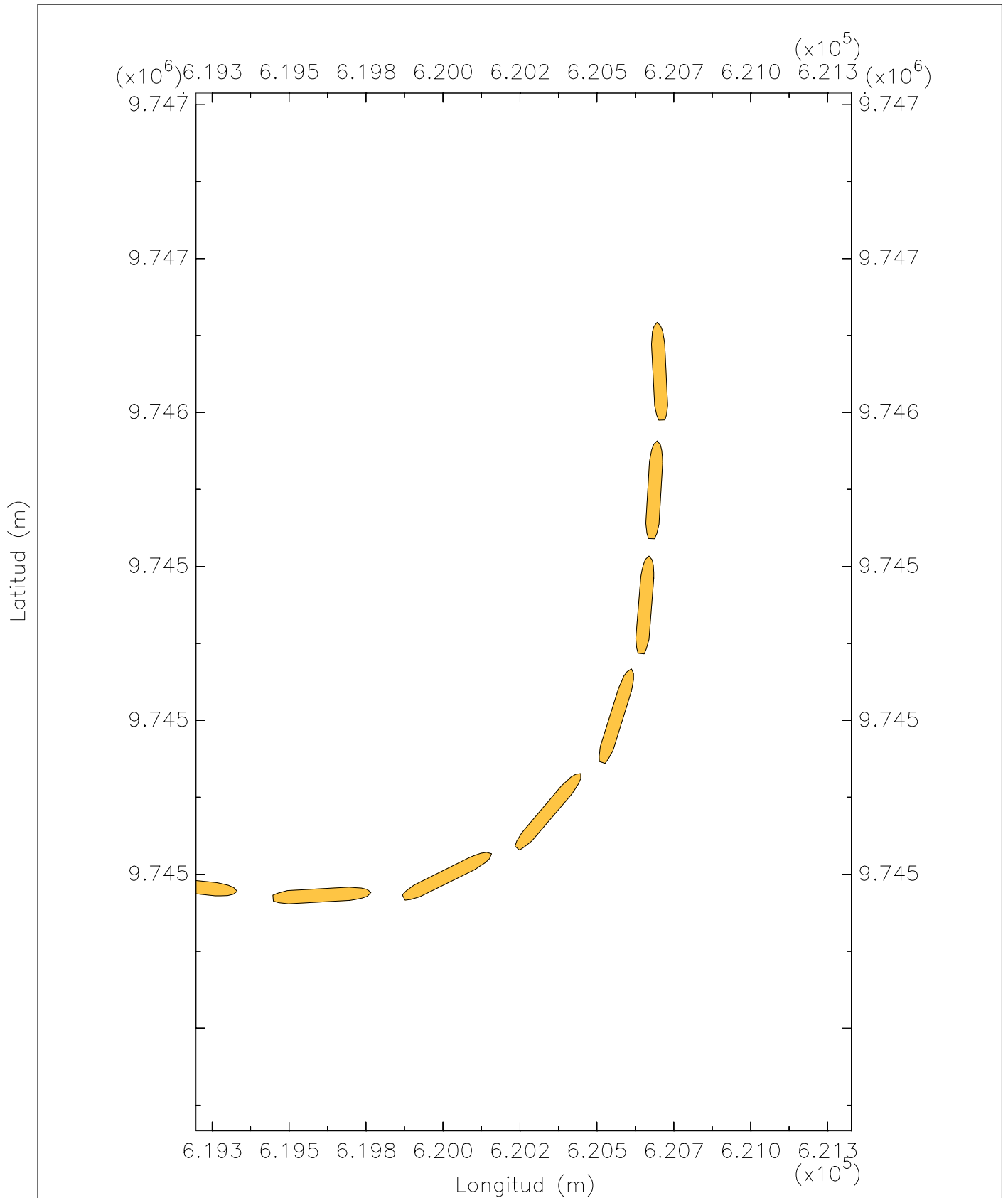
Z3T3 Trayectoria del barco portacontenedores post-panamax en flujo
