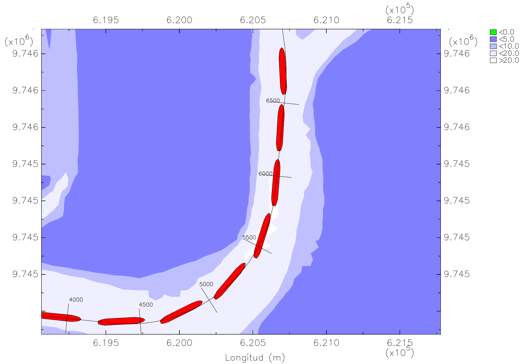
Z3T3 Trayectoria del barco portacontenedores post-panamax en flujo
