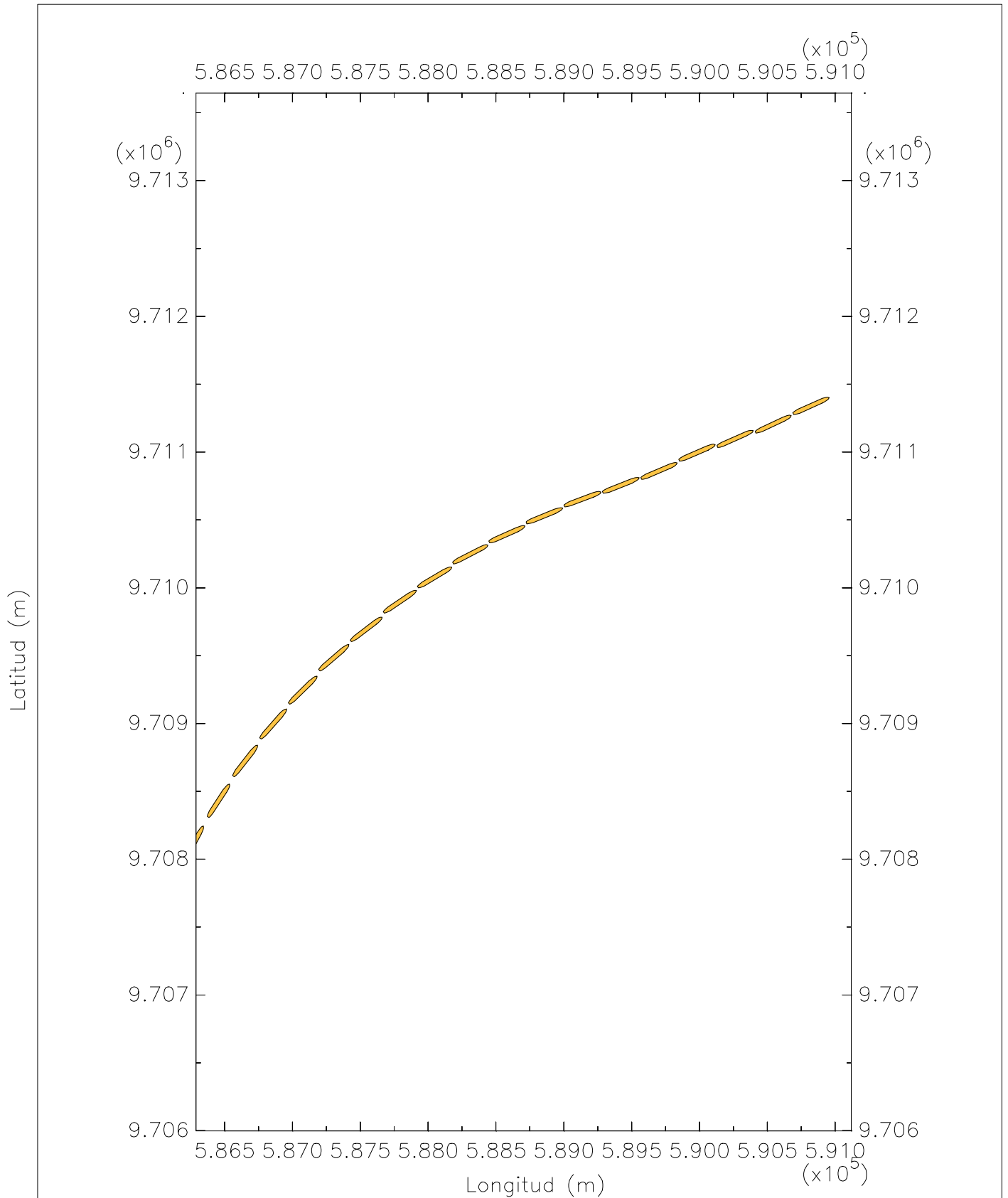
Z2T2 Trayectoria del barco panamax en flujo
