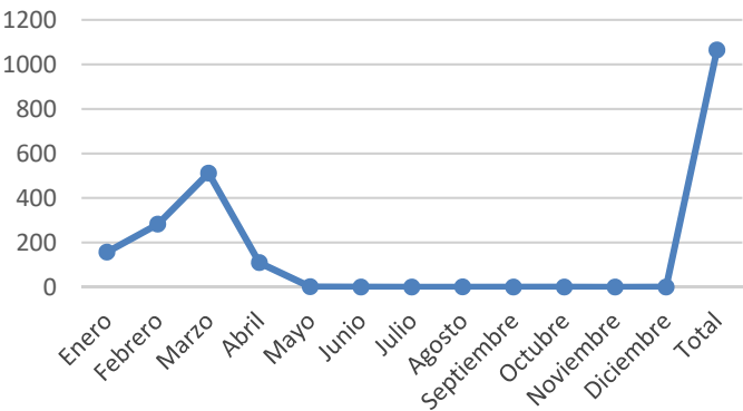
Ilustración 3.9. Precipitaciones
