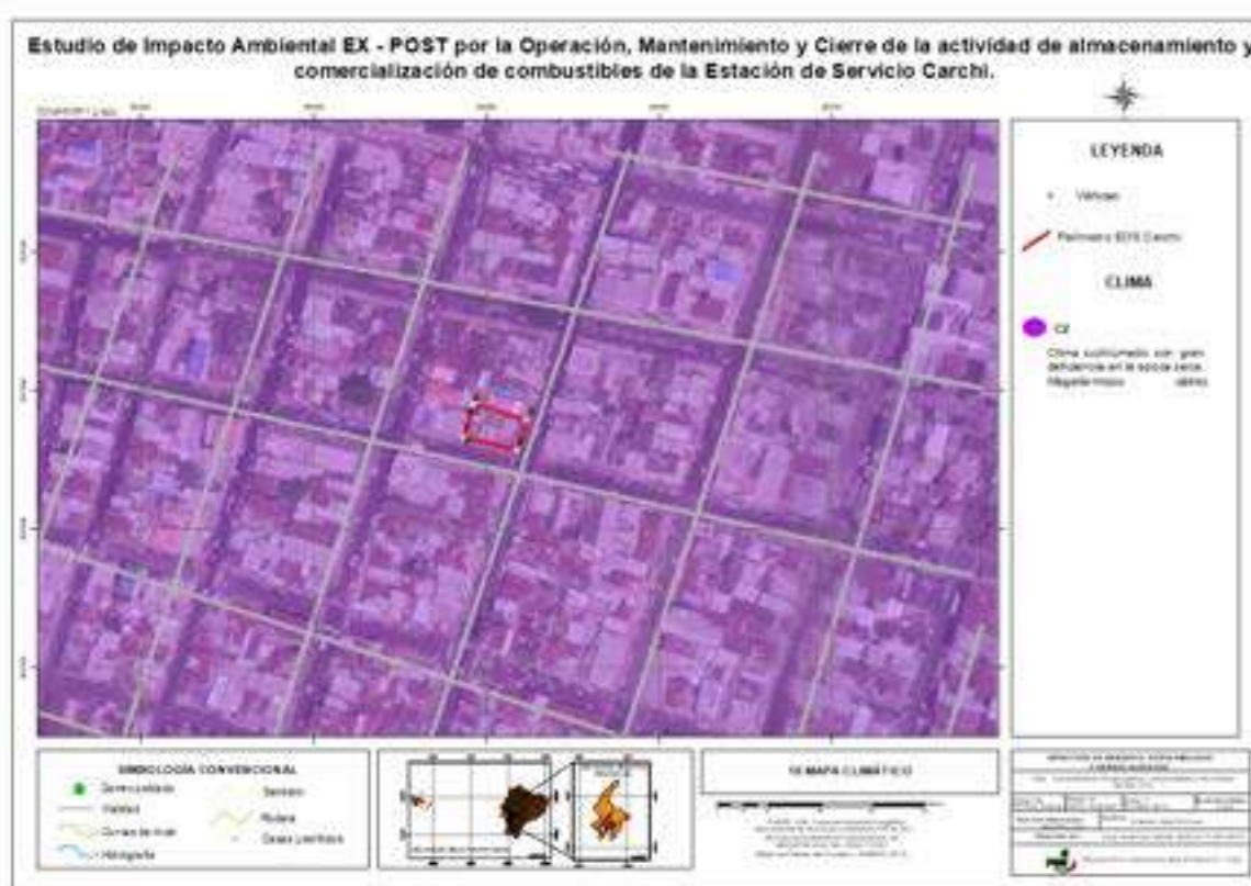
Ilustración 3.5. Mapa climático
